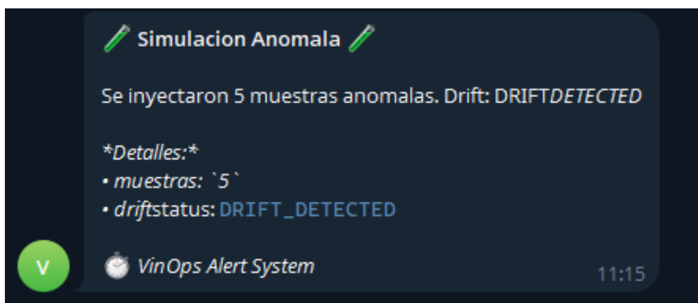
Figura 12: Alerta enviada por Telegram tras detectar comportamiento anómalo en el sistema monitorizado.
