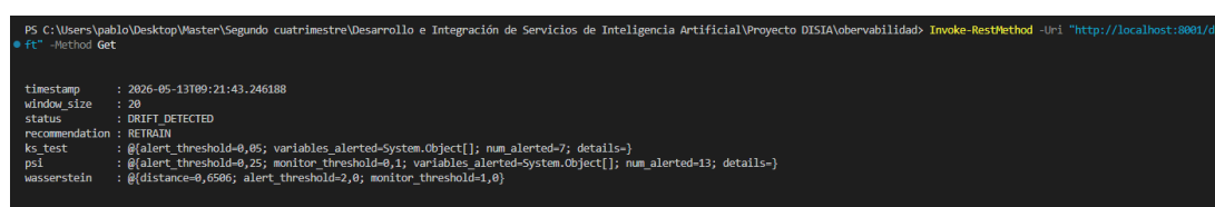
Figura 14: Estado de drift tras la simulación, mostrando activación del monitor y recomendación generada.
